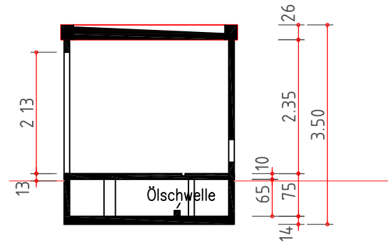
Längsschnitt A - A
