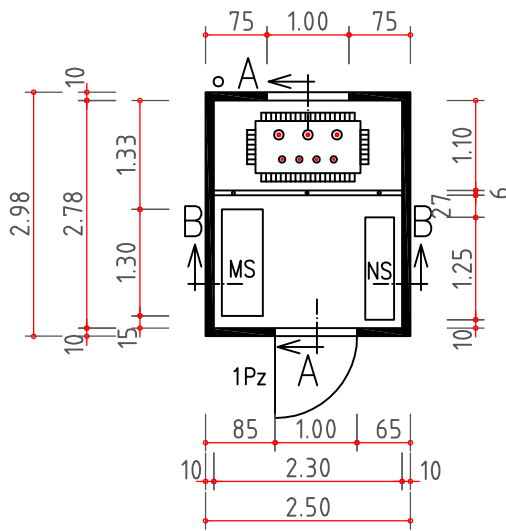
Grundriss
