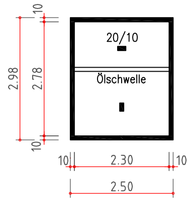
Kabelkeller
