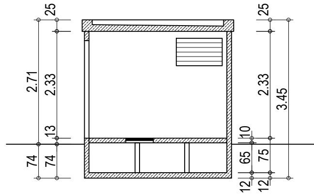
Längsschnitt A - A
