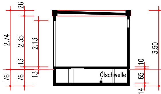
Längsschnitt A - A
