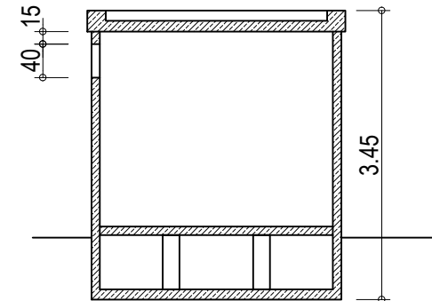
Querschnitt B - B
