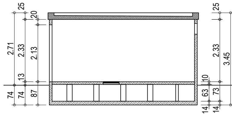
Längsschnitt A - A
