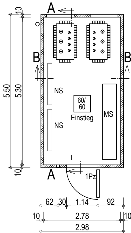
Grundriss
