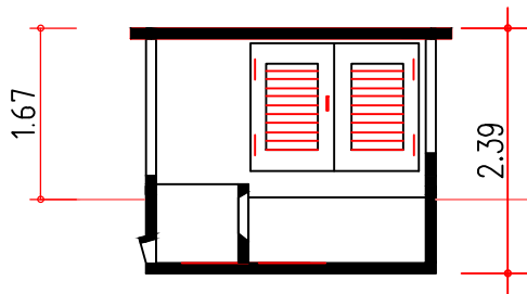
Längsschnitt
