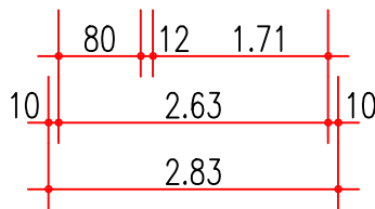
Grundriss
