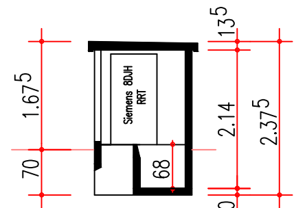
Querschnitt
